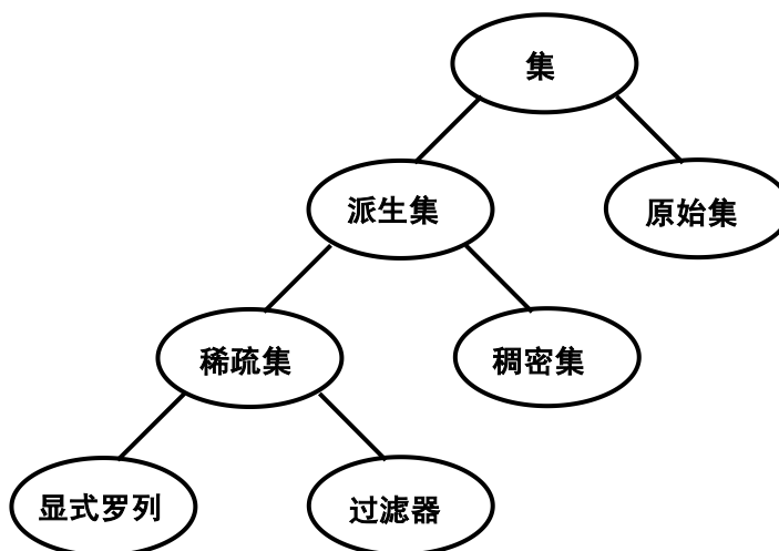
LINGO 集类型
