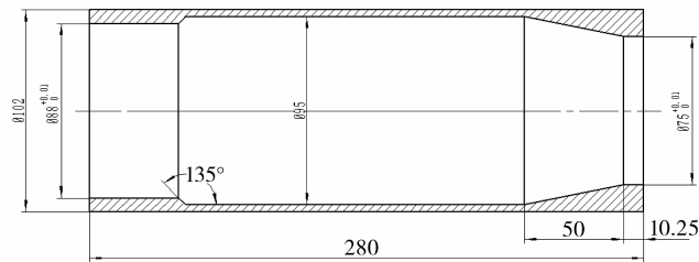
图 4 半成品图
