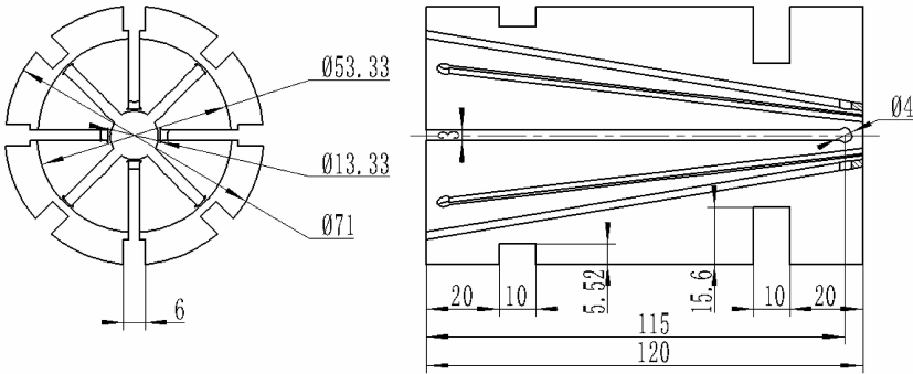
图 8 工件装夹图
