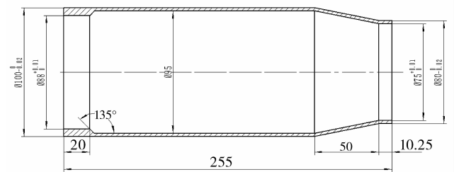
图 1 产品图
