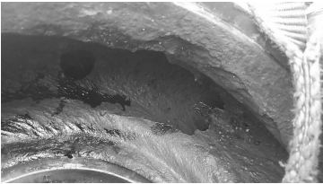
图 4 泵壳流道
