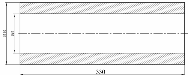
图 2 坯料图
