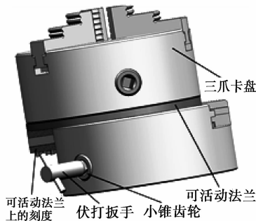
图 3 法兰驱动机构的工作原理
