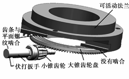
图 3 法兰驱动机构的工作原理
