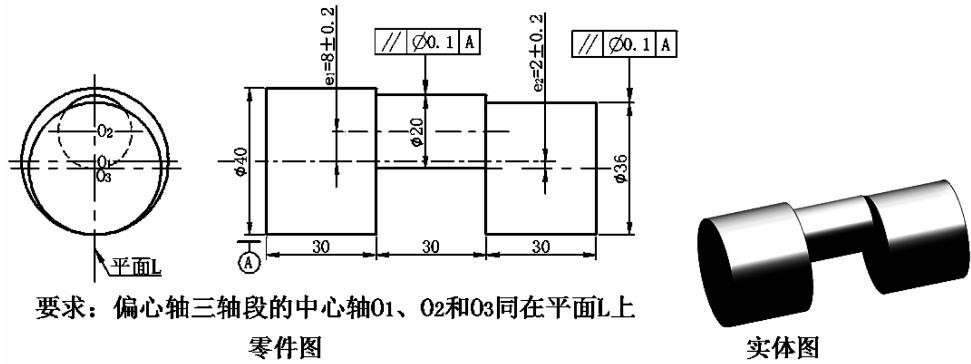
图 1 三轴段偏心的偏心轴
