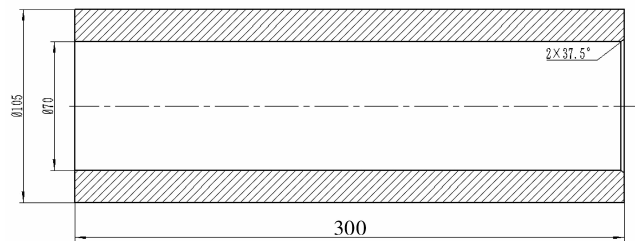
图 3 精坯料图
