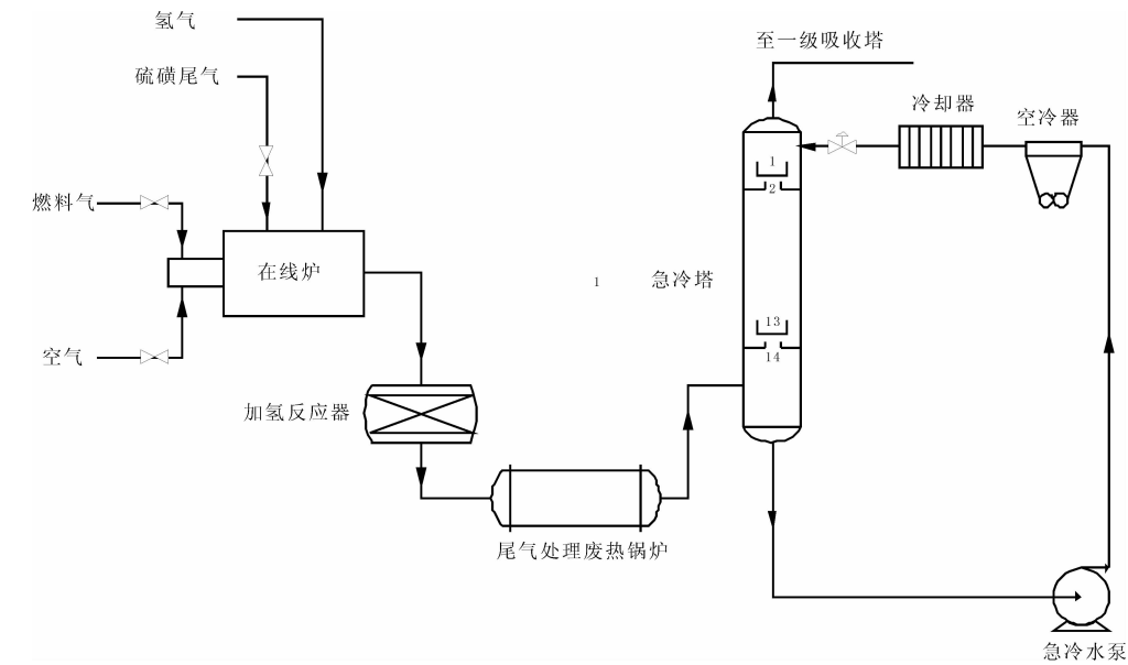
图 1 炼油厂尾气处理单元流程示意图
