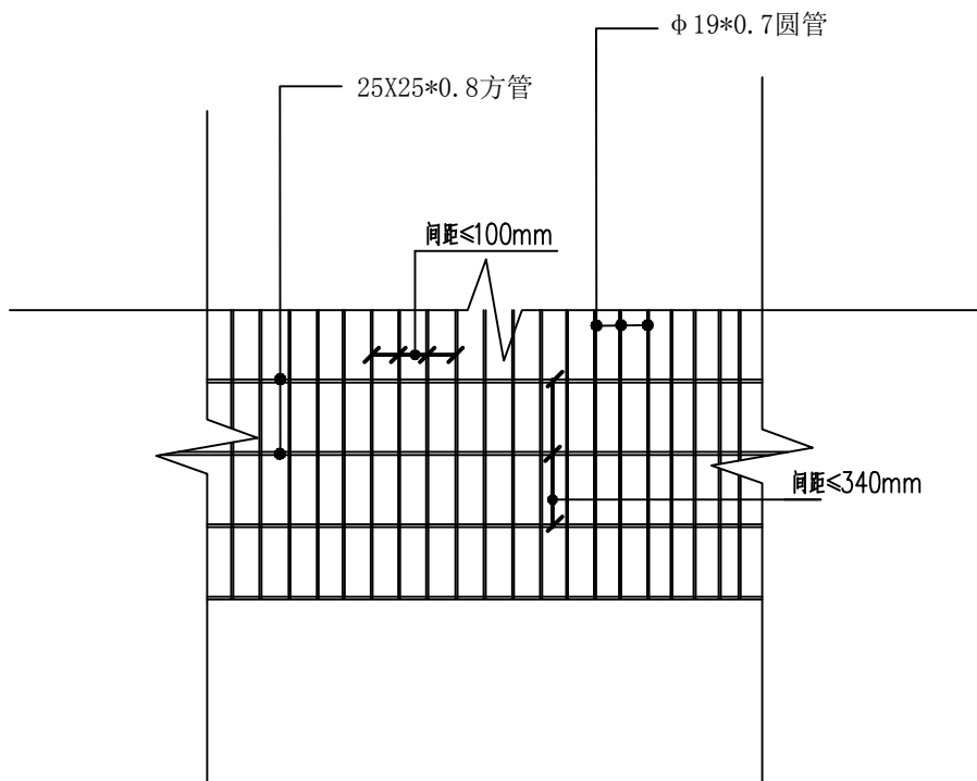
防盗网尺寸图
