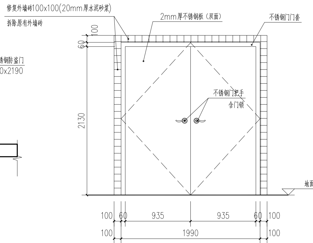
9号教学楼天台 更换门立面图 1:20
