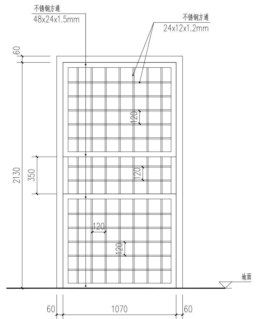
不锈钢门结构图 1:20
