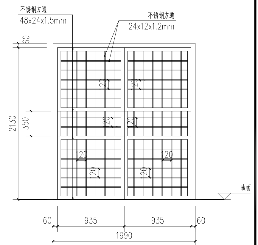
不锈钢门结构图 1:20
