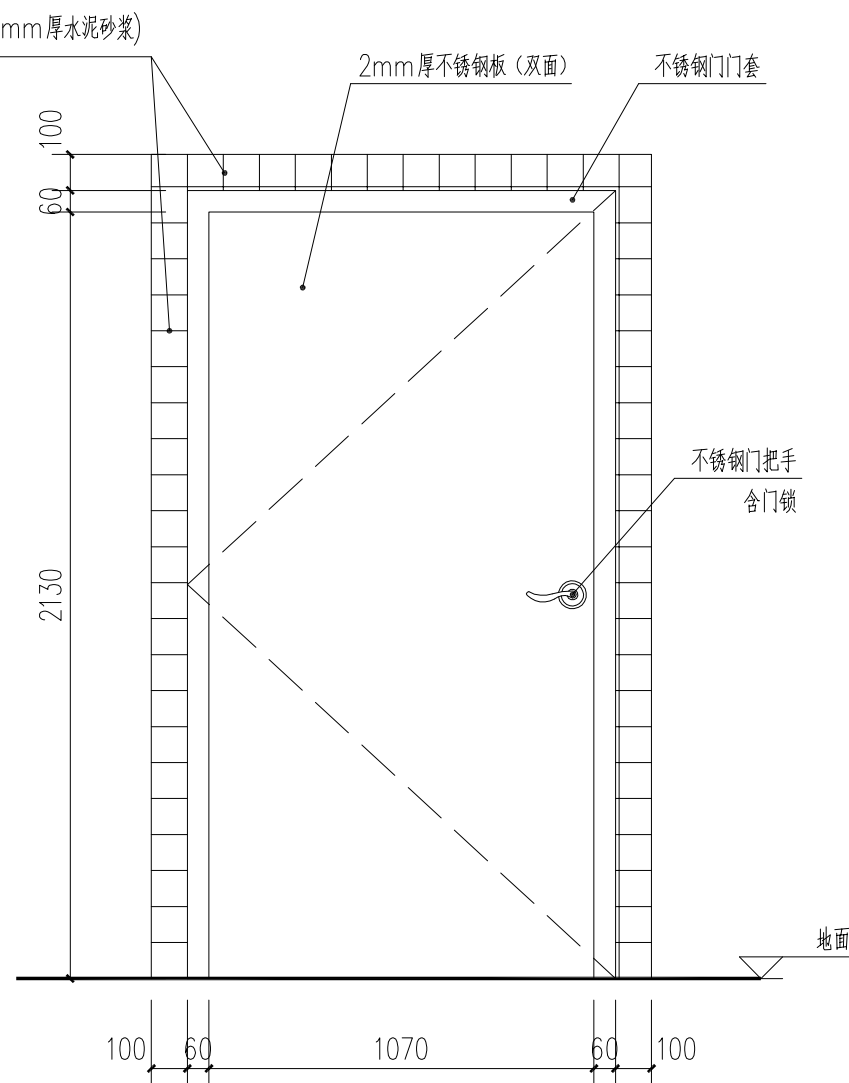
7号教学楼天台 更换门立面图 1:20
